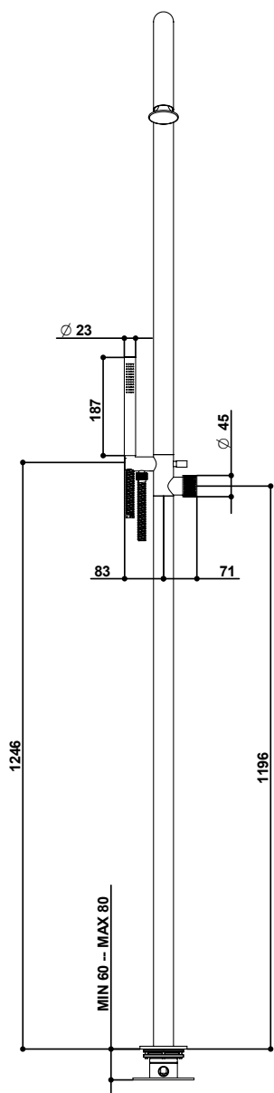
Corpo incasso Built-in body
