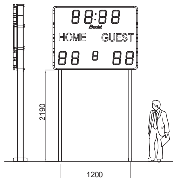
Support A BT 2025 P Classic Z1 to Z4
